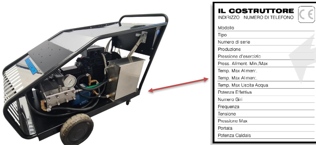
FIGURA 1 SECCIÓN 1.6 - Datos de marcado y placa de identificación de la máquina
